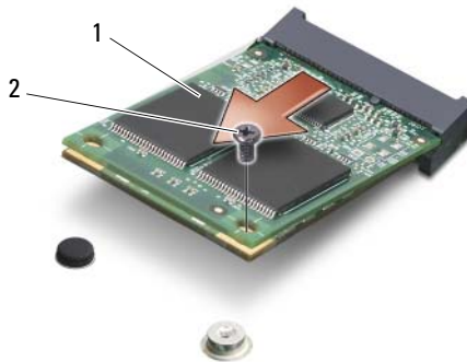
1 FCM-kaart 2 M2 x 3-mm schroef
