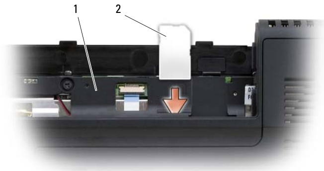
1 batterijcompartiment 2 SIM
